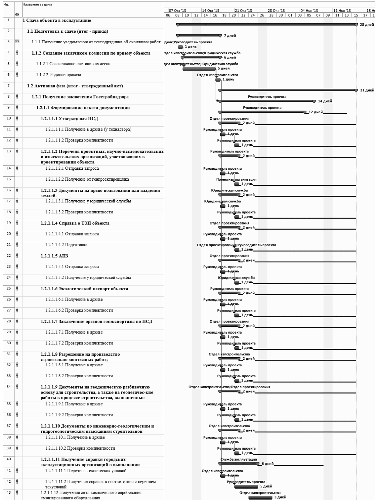
Рисунок 1 — Проект ввода в эксплуатацию объекта строительства
