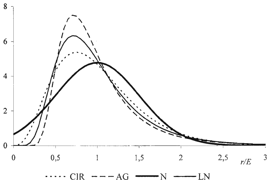
Рисунок 1 – Вид стационарных плотностей вероятностей для рассматриваемых моделей: Васичека (N), Блэка – Карасинского (LN), Кокса – Ингерсолла – Росса (CIR) и Ана – Гао (AG) для E^2/V = 4 .
