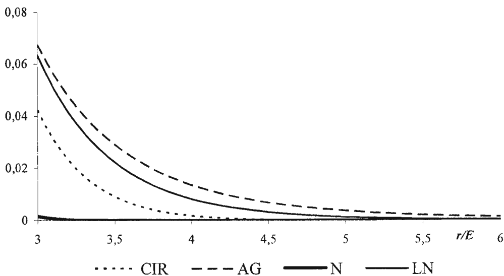
Рисунок 2 – Правые хвосты плотностей вероятностей, изображенных на рис. 1
