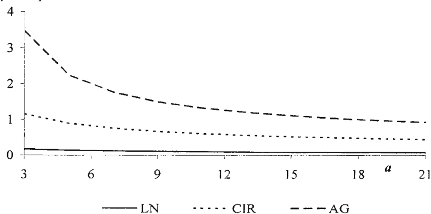
Рисунок 5 – Величина асимметрии как функция параметра a
