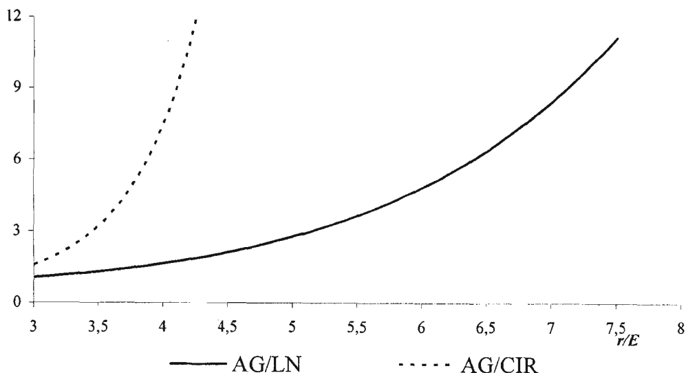
Рисунок 3 – Отношения плотностей вероятностей для моделей Ана – Гао (AG) и Блэка – Карасинского (LN), а также для моделей Ана – Гао (AG) и Кокса – Ингерсолла – Росса (CIR)
