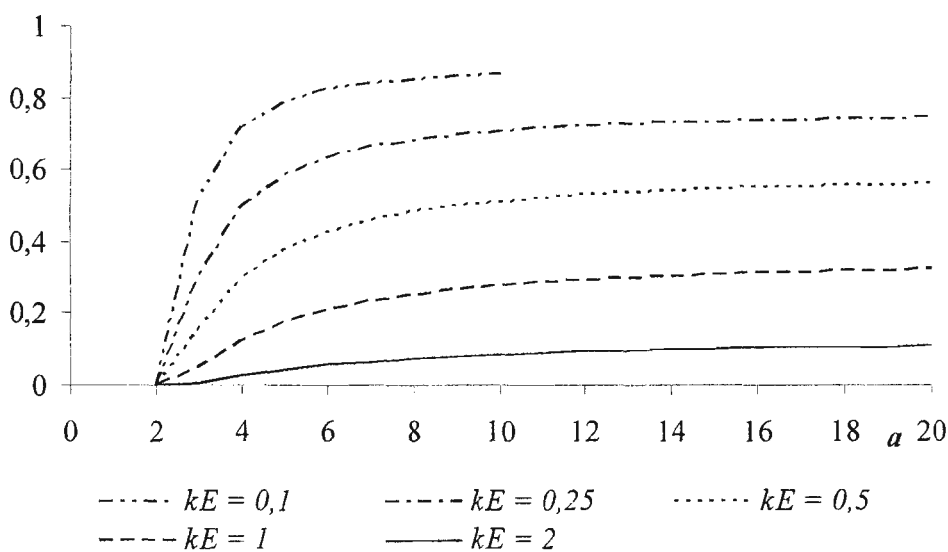
Рисунок 7 – Характер зависимости коэффициента корреляции от параметров kE и a при t_i - t_j = 1
