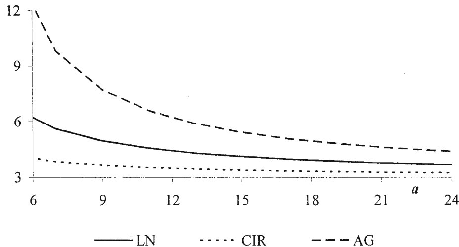
Рисунок 6 – Величина эксцесса как функция параметра a
