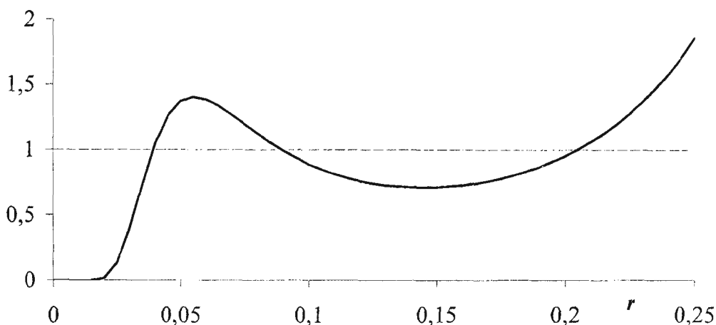
Рисунок 4 – Отношение h(r)/g(r) плотностей вероятностей h(r) и g(r) как функция переменной r для E = 0,08 и V = 0,0016
